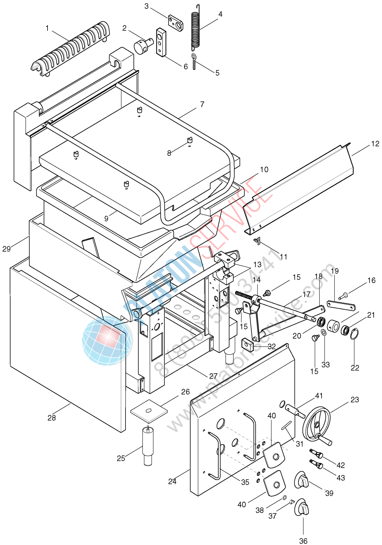
Brasiera Elettrica N700 Electric Bratt-Pan N700
